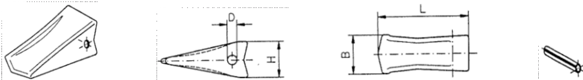
Flachkappe
