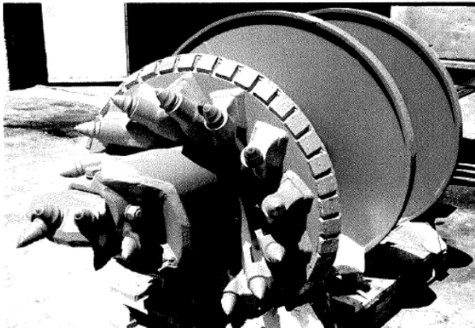
Progressivbohrschnecke
